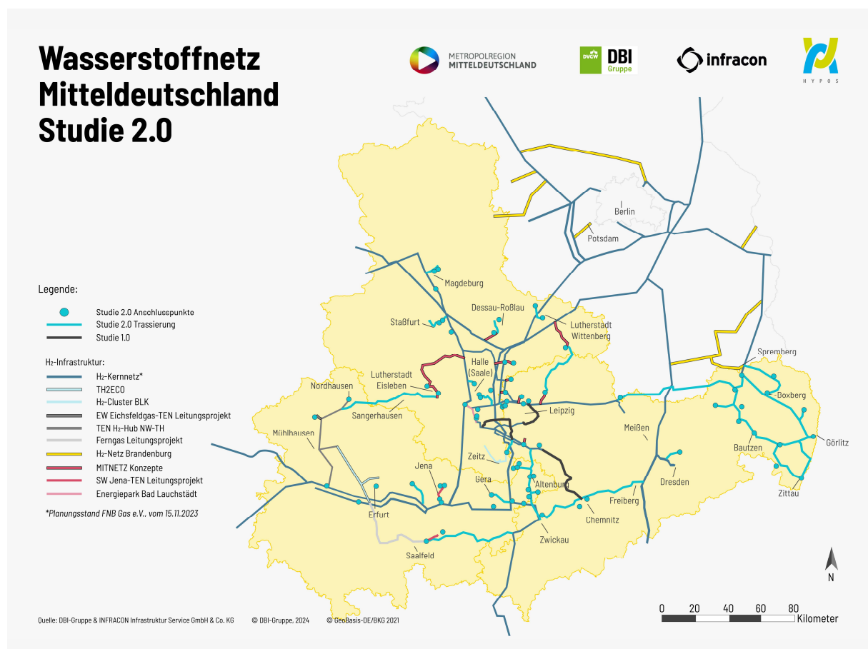
Abbildung 1: Trassierung des mitteldeutschen Wasserstoffnetzes der Studie 2.0
